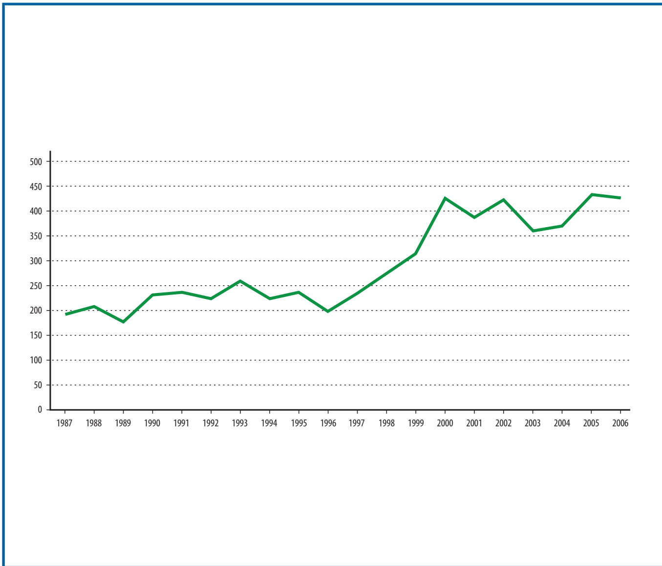
Source : Traduction libre. R. BELOW, D. GUHA-SAPIR, P. HOYOIS, J.-M. SCHEUREN, Centre for Research on the Epidemiology of Disasters (CRED), Université de Louvain, Belgique, Graphique extrait du document « Annual Disaster Statistical Review : Numbers and Trends », mai 2007, [en ligne]. (Consulté le 7 octobre 2008.)
